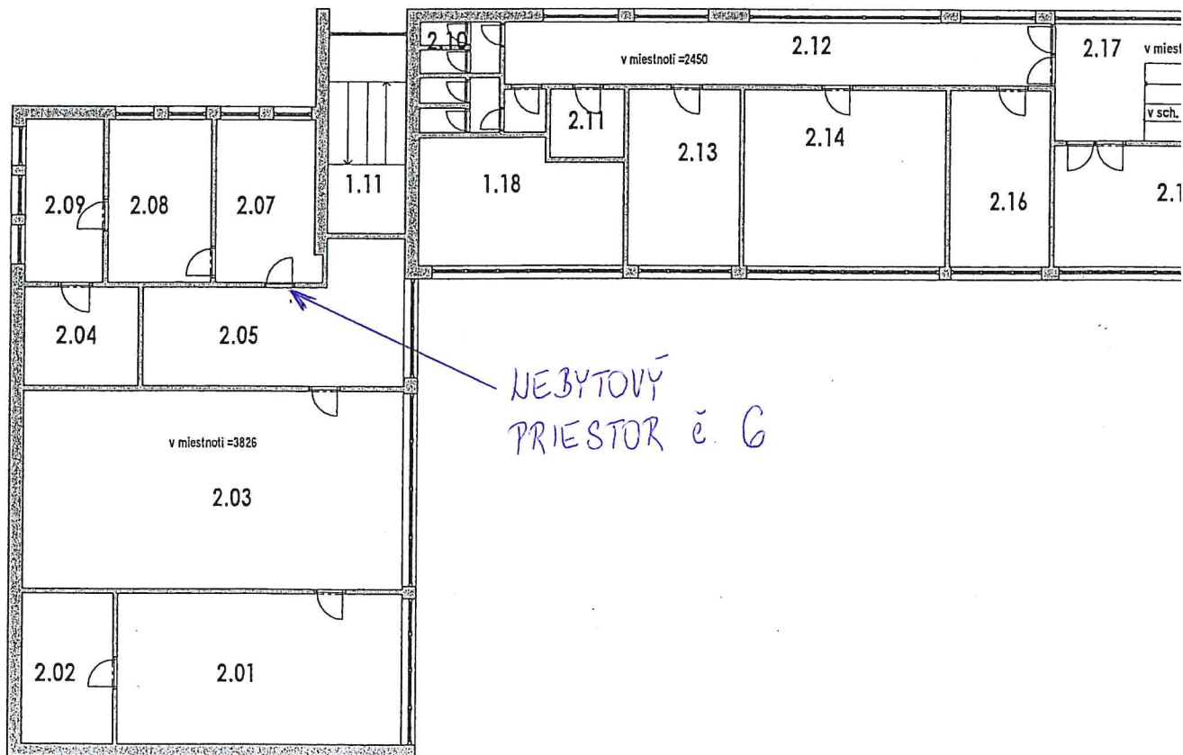
2 NP. PODLAŽIE 1 : 200
