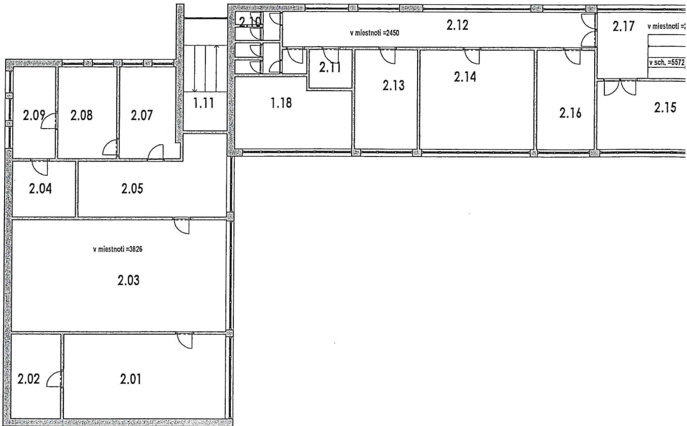
2 NP. PODLAŽIE 1 : 200
